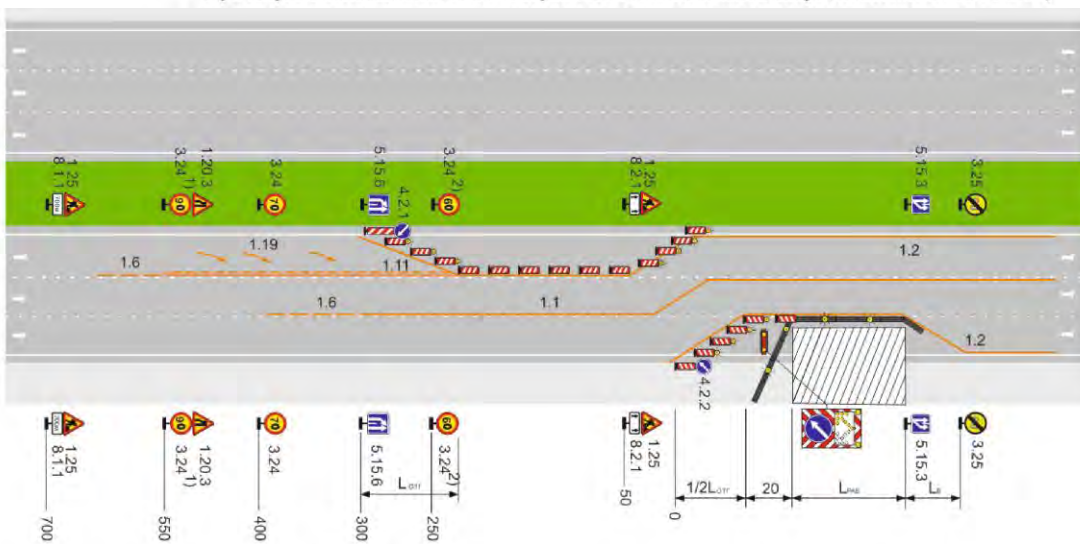
Рисунок Б.20 – Автомагистраль, скоростная дорога, шестиполосная дорога обычного типа. Рабочая зона производства долговременных работ на крайней правой полосе. Пропуск транспортных средств по двум полосам с предварительным изменением траектории движения
