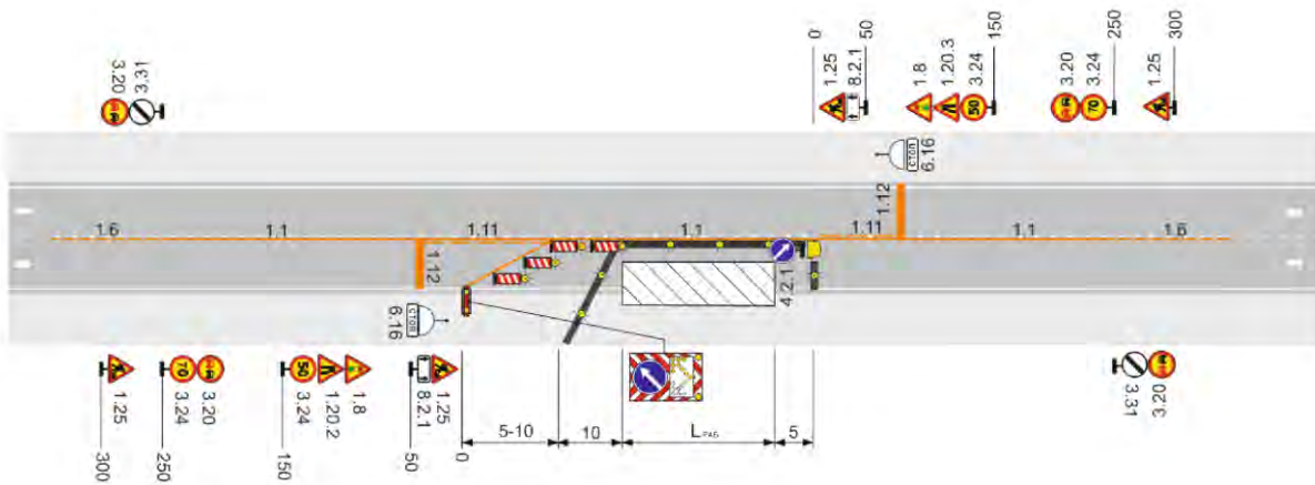
Рисунок Б.2 – Двухполосная дорога. Рабочая зона производства долговременных работ на полосе движения на подъем. Пропуск транспортных средств встречных направлений по одной полосе с помощью дорожных знаков (интенсивность движения менее 250 авт./ч в двух направлениях)
