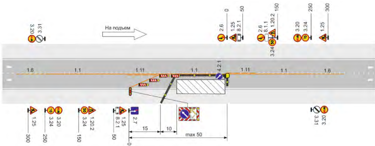
Рисунок Б.2 – Двухполосная дорога. Рабочая зона производства долговременных работ на полосе движения на подъем. Пропуск транспортных средств встречных направлений по одной полосе с помощью дорожных знаков (интенсивность движения менее 250 авт./ч в двух направлениях)
