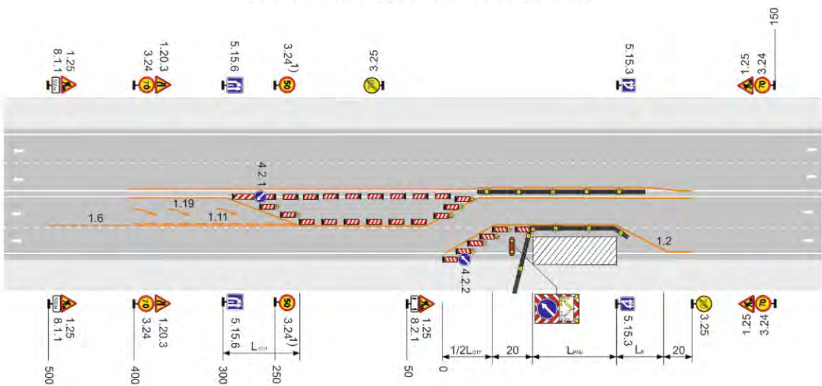
Рисунок Б.18 – Четырехполосная дорога обычного типа без разделительной полосы. Рабочая зона производства долговременных работ на крайней правой полосе движения. Пропуск транспортных средств по одной полосе с предварительным изменением траектории движения
