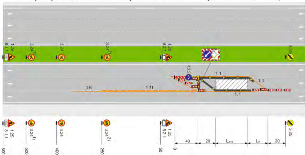
Рисунок Б.23 – Автомагистраль, скоростная дорога, шестиполосная дорога обычного типа. Рабочая зона производства долговременных работ на крайней левой и средней полосах движения. Пропуск транспортных средств по одной полосе и обочине. 1 На дороге обычного типа знак не ставится. 2 При ширине полосы движения 3 м ограничение максимальной скорости движения до 50 км/ч)
