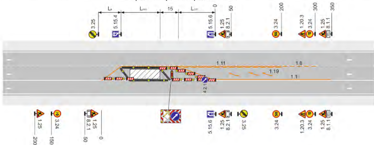
Рисунок Б.14 – Трехполосная дорога. Рабочая зона производства долговременных работ на крайней полосе движения. Пропуск транспортных средств по крайней и средней полосам
