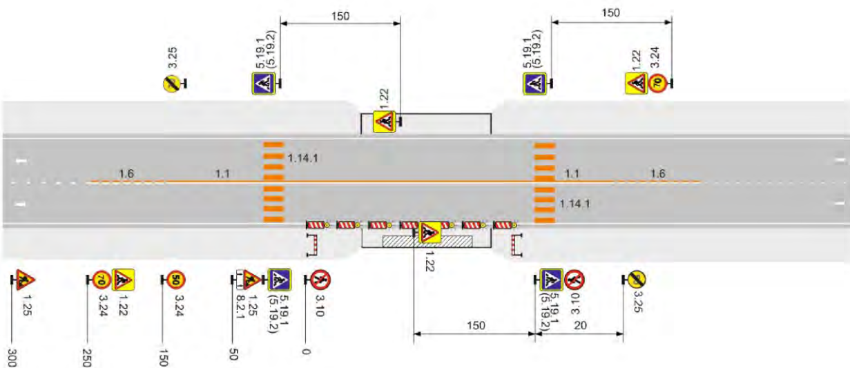
Рисунок Б.8 – Двухполосная дорога. Рабочая зона производства долговременных работ на полосе движения и тротуаре моста (путепровода). Пропуск транспортных средств встречных направлений по одной полосе с помощью светофорного регулирования
