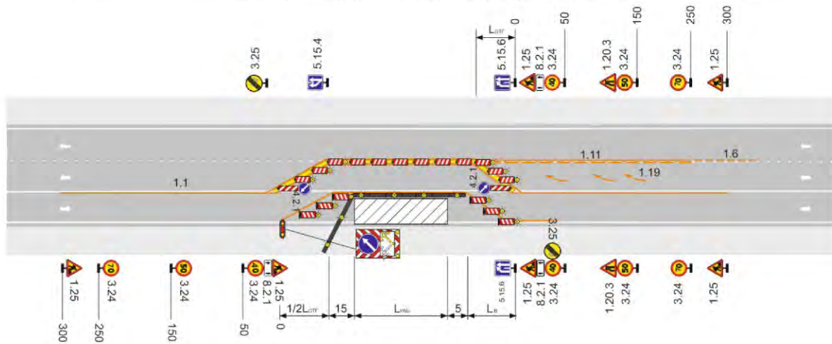
Рисунок Б.13 – Двухполосная дорога. Рабочая зона производства долговременных работ на всей ширине проезжей части. Пропуск транспортных средств в объезд по существующим дорогам
