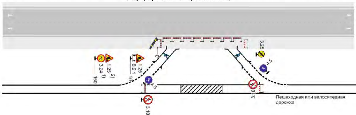
Рисунок Б.6 – Двухполосная дорога. Рабочая зона производства долговременных работ на обочине или откосе с сужением полосы движения (1) При разрытии блоки парпетного типа
