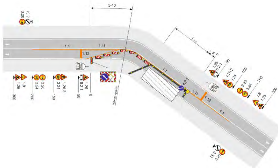
Рисунок Б.3 – Двухполосная дорога. Рабочая зона производства долговременных работ на полосе движения. Пропуск транспортных средств встречных направлений по одной полосе с помощью светофорного регулирования
