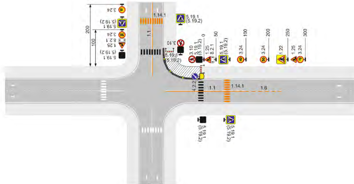
Рисунок Б.11 – Двухполосная дорога. Рабочая зона производства долговременных работ на пересечении в одном уровне на всей ширине проезжей части. Пропуск транспортных средств по обочинам
