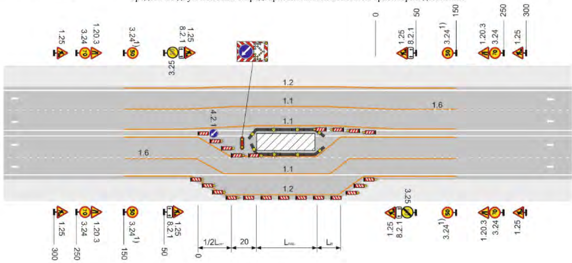
Рисунок Б.16 – Трехполосная дорога. Рабочая зона производства долговременных работ на крайней полосе движения. Пропуск транспортных средств по двум полосам с предварительным изменением траектории движения
