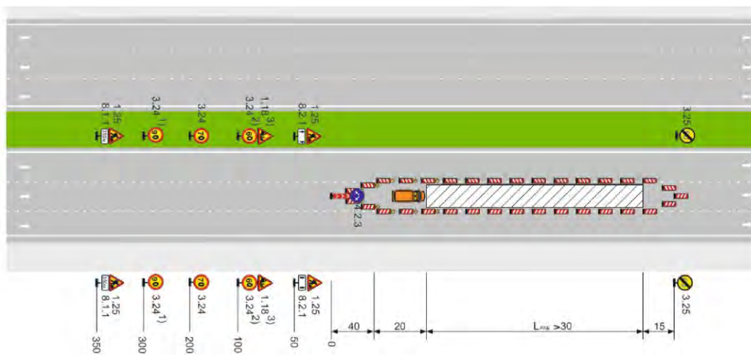
Рисунок Б.40 – Автомагистраль, скоростная дорога, многополосная дорога обычного типа с разделительной полосой. Рабочая зона производства краткосрочных работ на средней полосе (полосах). Пропуск транспортных средств по существующим свободным полосам
