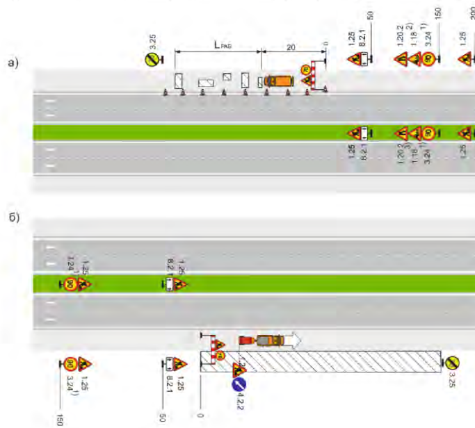
Рисунок Б.37 – Автомагистраль, скоростная дорога, многополосная дорога обычного типа. Рабочая зона производства краткосрочных работ на обочине (а) или откосе (б)
