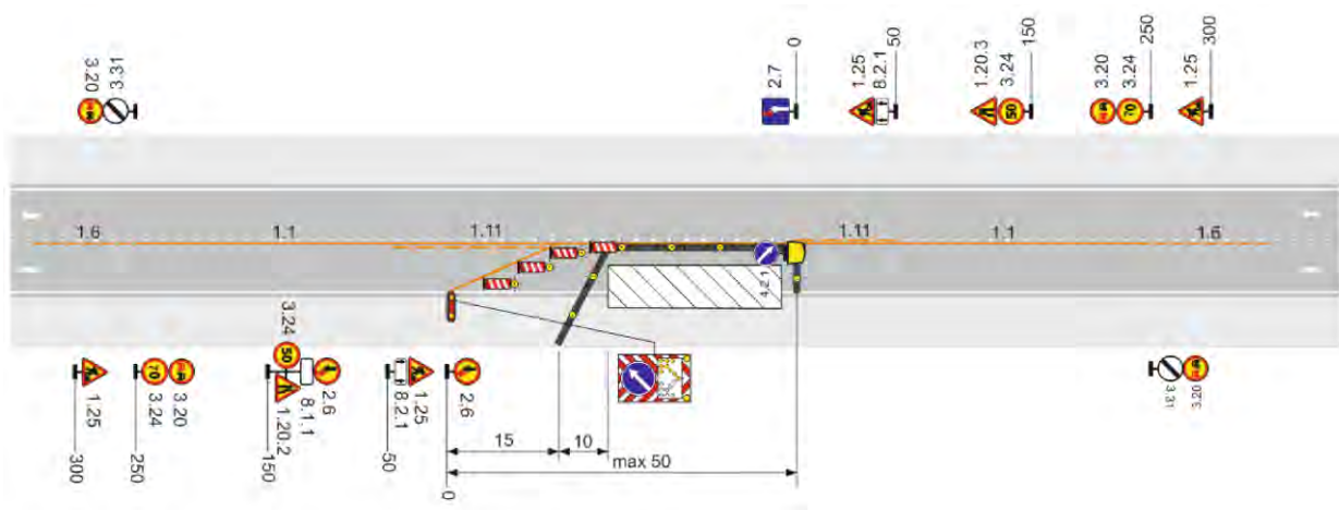
Рисунок Б. 1 – Двухполосная дорога. Рабочая зона производства долговременных работ на полосе движения. Пропуск транспортных средств встречных направлений по одной полосе с помощью дорожных знаков (интенсивность движения менее 250 авт./ч в двух направлениях)
