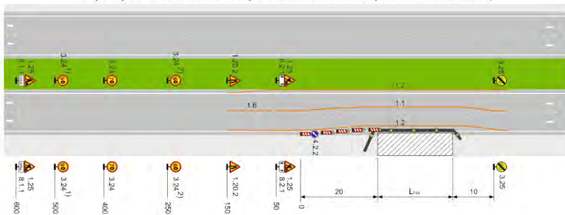
Рисунок Б.25 – Автомагистраль, скоростная дорога, многополосная дорога обычного типа. Рабочая зона производства долговременных работ на обочине или откосе. Пропуск транспортных средств по существующим полосам с уменьшением ширины крайней правой полосы 1) На дороге обычного типа знак не ставится. 2) При ширине полосы движения 3 м ограничение максимальной скорости движения до 50 км/ч)
