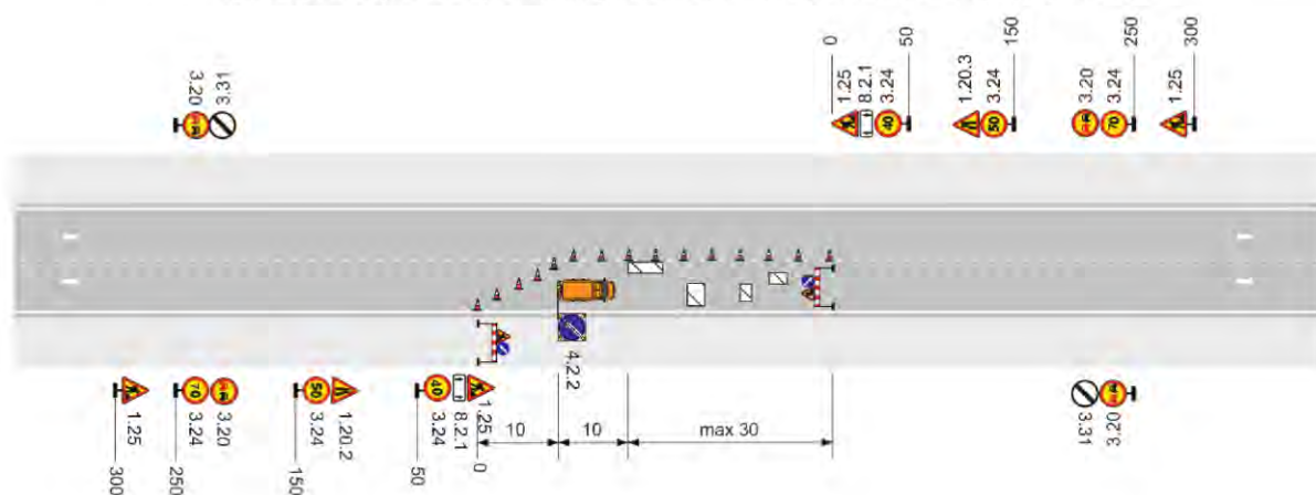
Рисунок Б.33 – Двухполосная дорога. Рабочая зона производства краткосрочных работ длиной более 30 м на полосе движения. Пропуск транспортных средств встречных направлений по одной полосе с помощью регулировщиков
