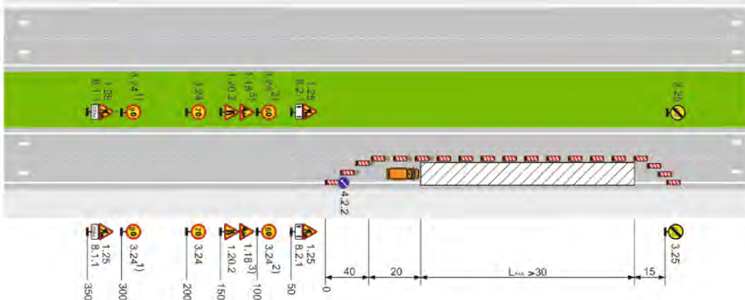
Рисунок Б.41 – Автомагистраль, скоростная дорога, многополосная дорога обычного типа с разделительной полосой. Рабочая зона производства краткосрочных работ на крайней правой полосе. Пропуск транспортных средств по существующим свободным полосам
