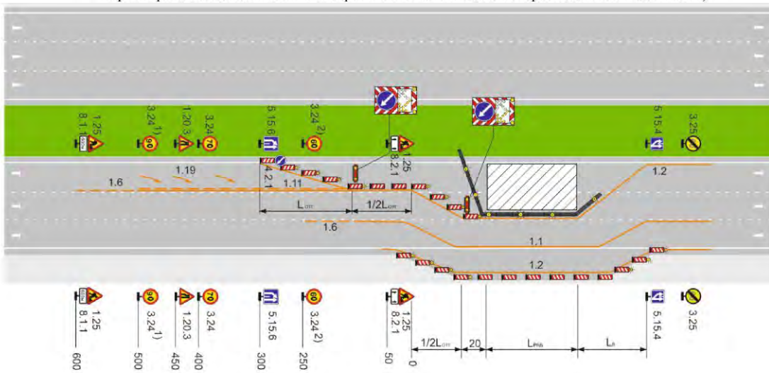
Рисунок Б.22 – Автомагистраль, скоростная дорога, четырехполосная дорога обычного типа с разделительной полосой. Рабочая зона производства долговременных работ на крайней левой полосе. Пропуск транспортных средств по одной полосе и обочине. 1 На дороге обычного типа знак не ставится. 2 При ширине полосы движения 3 м ограничение максимальной скорости движения до 50 км/ч)
