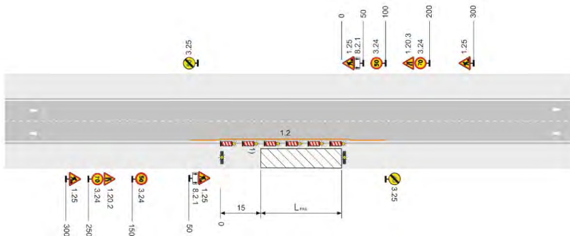
Рисунок Б.5 – Двухполосная дорога. Рабочая зона производства долговременных работ на полосе движения. Пропуск транспортных средств по полосе встречного движения и обочине
